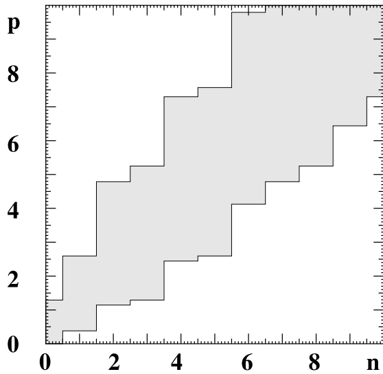
Рис. 6: Доверительная зона для оценки параметра p распределения Пуассона с уровнем доверия \beta = 0.6827
