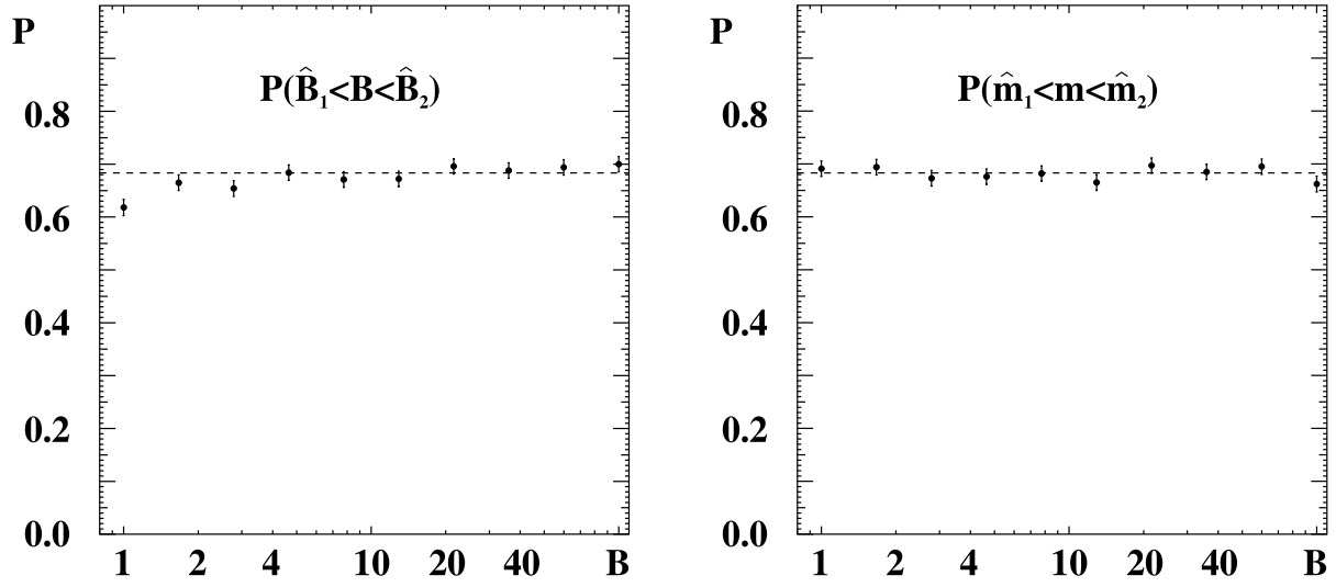
Рис. 13: Вероятность покрытия истинных значений параметров B и m резонансной кривой доверительными интервалами (\hat{B}_1, \hat{B}_2) и (\hat{m}_1, \hat{m}_2) , соответственно, полученными по функции правдоподобия на уровне \Delta L = 1/2 (ожидаемый уровень доверия 68%). Статистика расчетов методом Монте-Карло в каждой точке — 10^3 “экспериментов”
