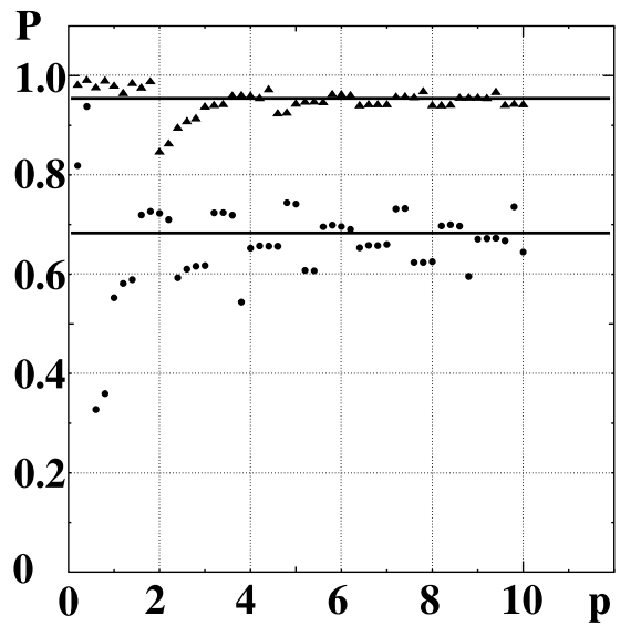
Рис. 5: Вероятность P попадания истинного значения параметра p Пуассонова распределения в доверительный интервал, полученный методом максимального правдоподобия. \bullet — 68%-ый доверительный интервал, \blacktriangle — 95%-ый доверительный интервал. Горизонтальные сплошные линии показывают “правильное” значение вероятности (0.6827 и 0.9545).
