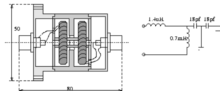
Рис. 5. Трансформатор
