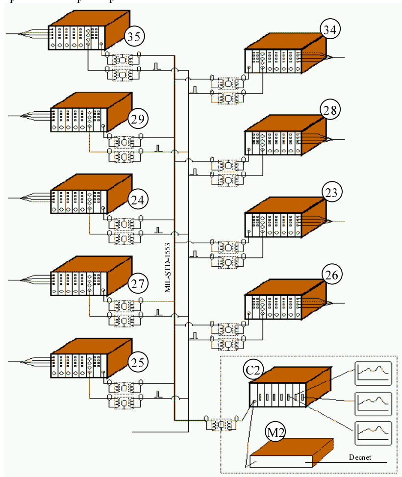
Рис. 3. Структура диагностического комплекса
