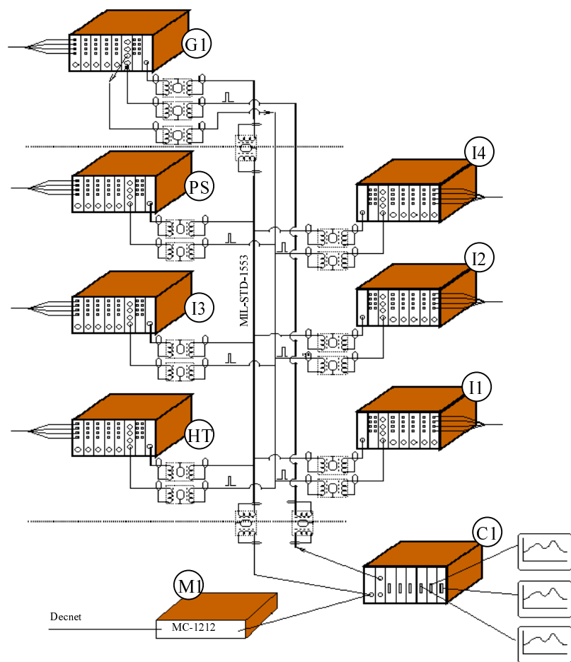
Рис. 2. Структура управляющего комплекса
